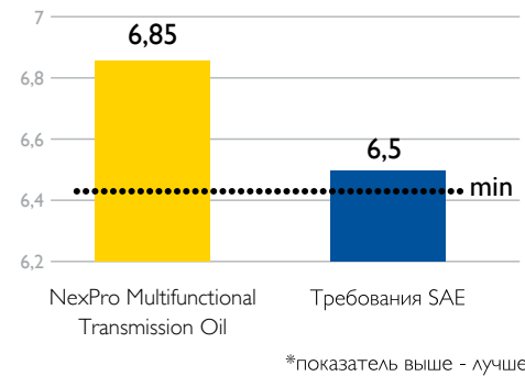
KRL-испытание в течение 100ч. по методу CEC-L-45-A-99*
