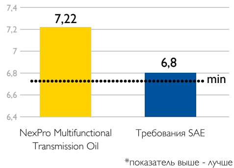
KRL-испытание в течение 20ч. по методу CEC-L-45-A-99*
