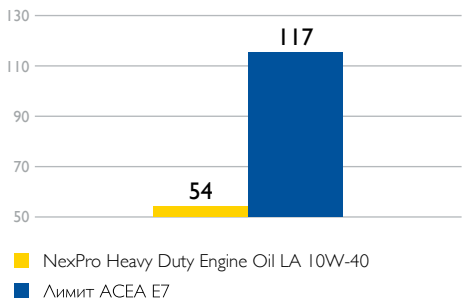
Износ поршневого кольца в тесте Mack T-12, мкм*
