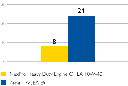
Потеря массы подшипников в тесте Mack T-12, мг*
